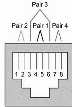
T568B
