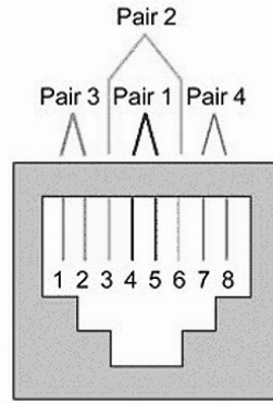
T568A
